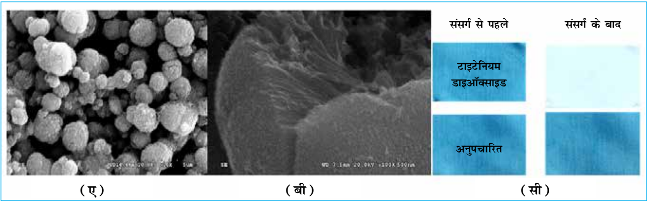
चित्र 4 : (ए) टाइटेनिया सूक्ष्मगोलकों की इलेक्ट्रॉन माइक्रोस्कोप इमेज (बी) सूक्ष्मगोलकों में व्यवस्थित रूप से मौजूद टाइटेनिया नैनोरोड, (सी) टाइटेनिया सूक्ष्मगोलकों की 'अपने-आप सफाई' की सुविधा को सूती कपड़े में मेथिलीन ब्लू रंग के साथ इस्तेमाल किया जाता है और इसके तहत कपड़े को 8 घंटे तक धूप में रखा जाता है। कपड़े के रंग में ज्यादा बदलाव नहीं होता। हालांकि, टीआईओ 2 से लैस कपड़ा मेथिलीन ब्लू को हल्का कर देता है और कपड़े का रंग खत्म कर देता है।
